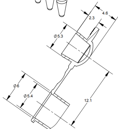
DETAIL B SCALE: 3.8 : 1 TYP
